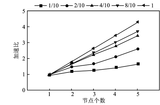
图 2 加速比实验结果
