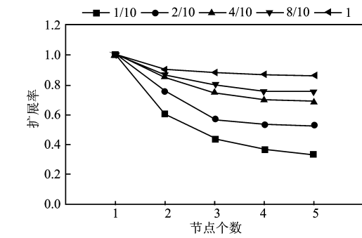
图 3 集群扩展性对比图
